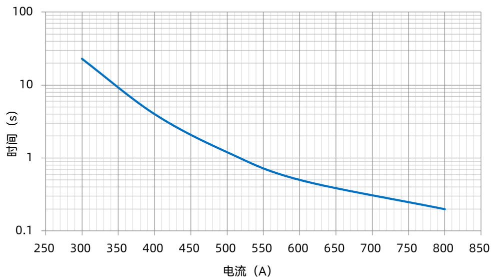
电流-时间曲线
